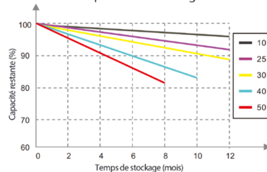
Caractéristiques d'auto-décharge
