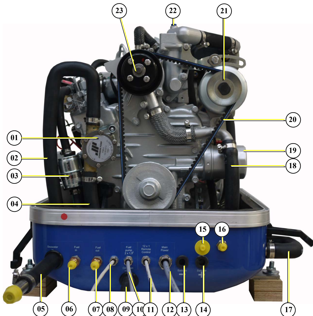
Fig. D.2.3-1: Vue frontale
