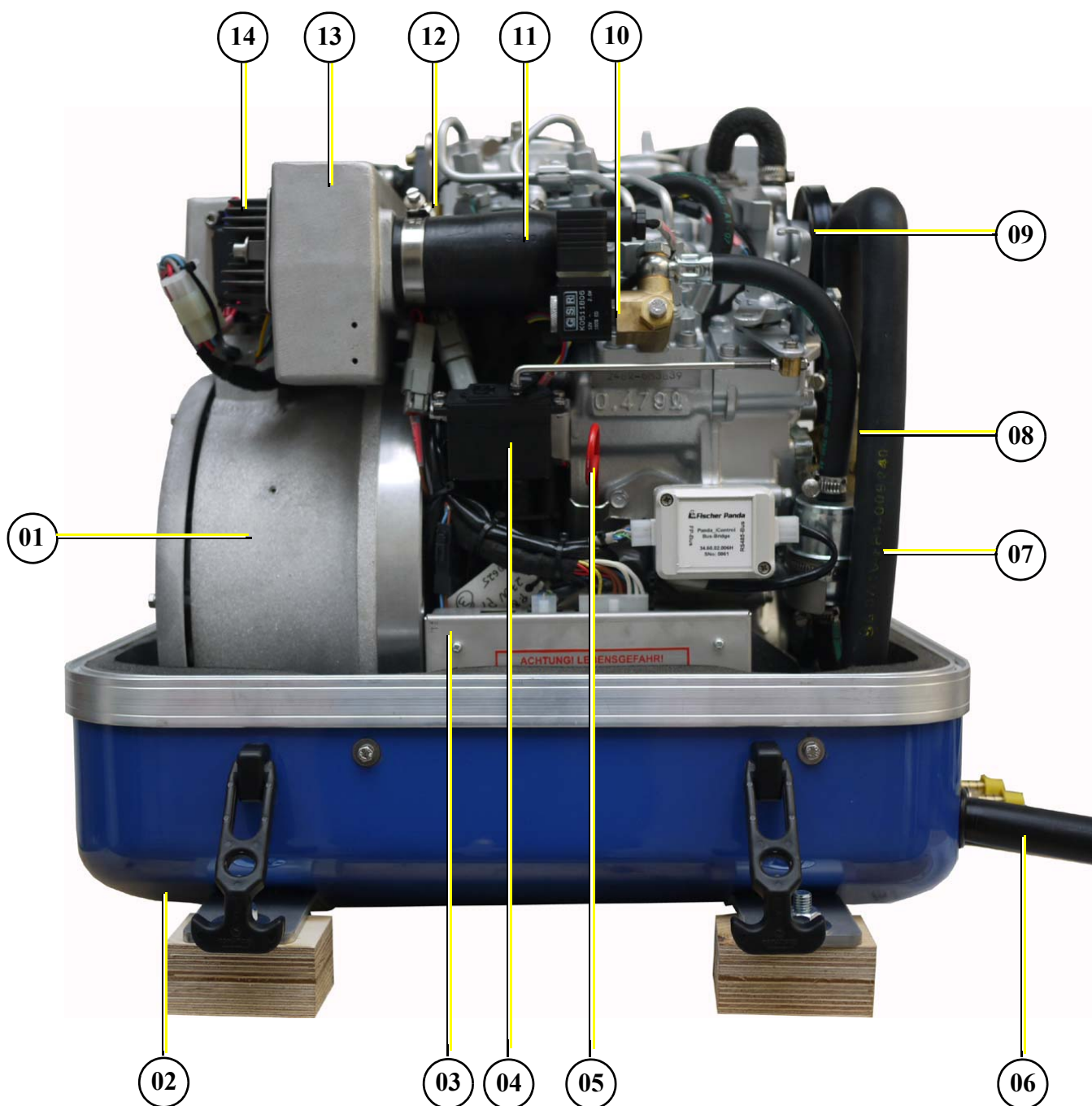
Fig. D.2.2-1: Vue latérale gauche
