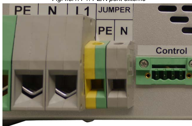
Fig. I.5.1.4-1: PE/N pont externe
