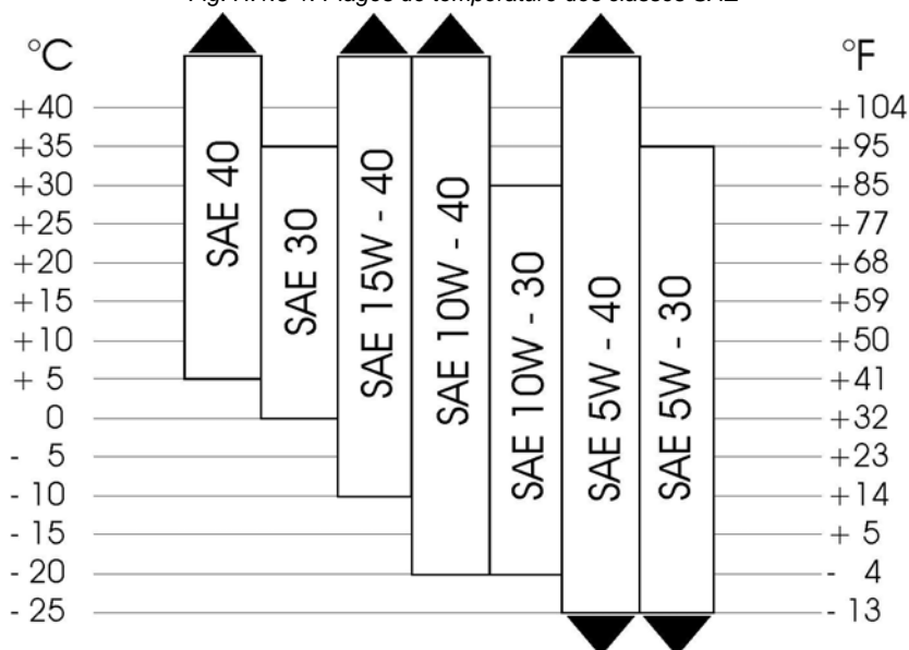
Fig. H.1.5-1: Plages de température des classes SAE
