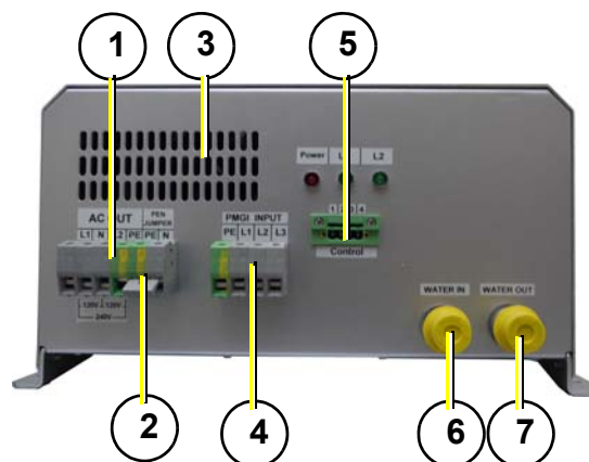
Fig. I.5-1: Côté raccordement
