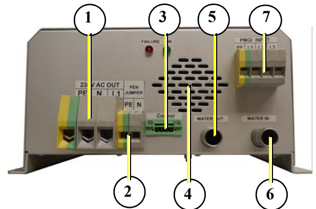
Fig. I.3-1: Côté raccordement
