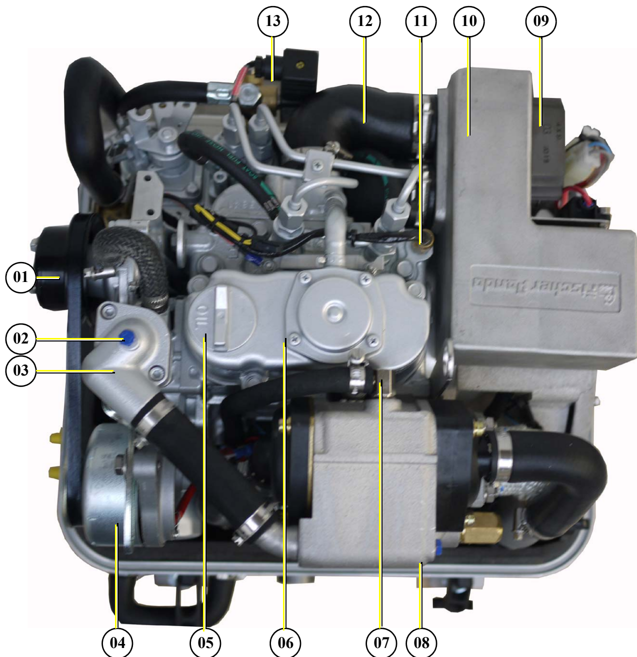
Fig. D.2.5-1: Vue de dessus
