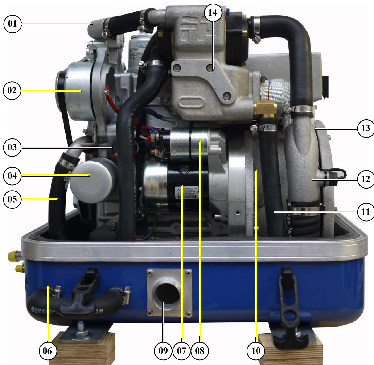
Fig. D.2.1-1: Vue latérale droite
