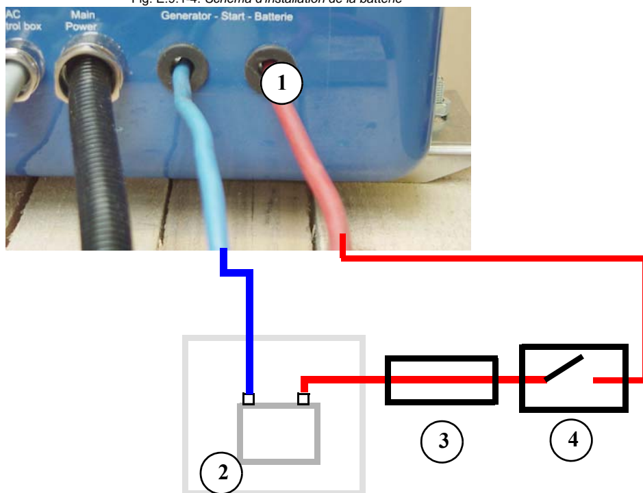
Fig. E.9.1-4: Schéma d'installation de la batterie
