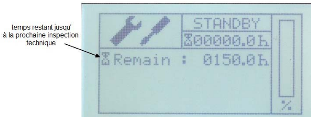
Fig. K.3.3.1-1: Page des infos service
