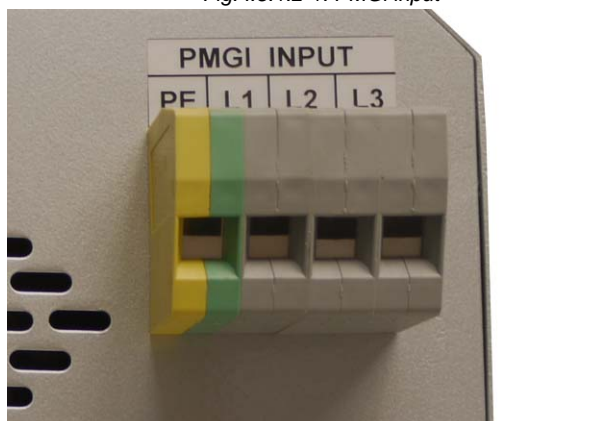
Fig. I.5.1.2-1: PMGi input
