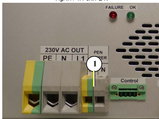
Fig. I.11-1: Pont PE-N
