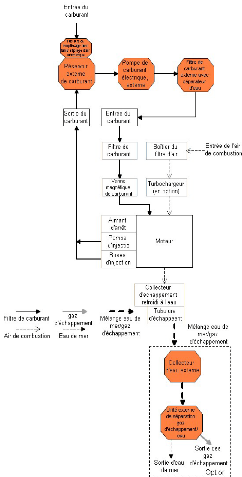
Fig. D.3.3-1: Système de combustion de carburant et d'échappement de gaz brûlés
