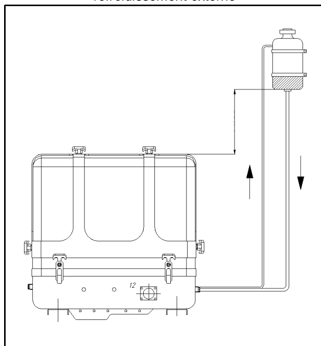
Fig. E.5.1-1: Position du bac d'expansion d'eau de refroidissement externe
