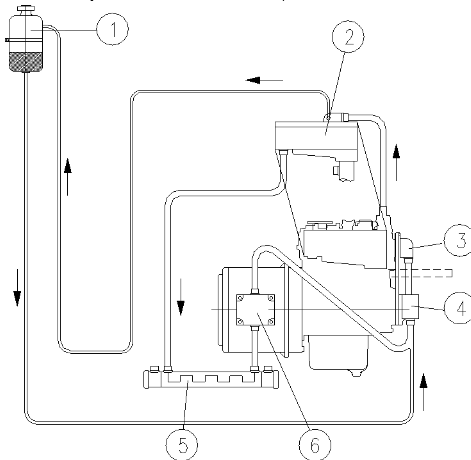
Fig. E.5.4-1: Schéma du circuit d'eau douce du système à deux circuits
