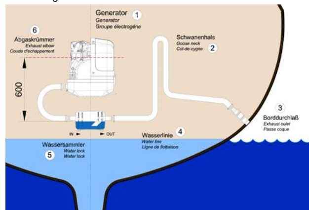
Fig. E.6.5.1-1: Position idéale du collecteur d'eau
