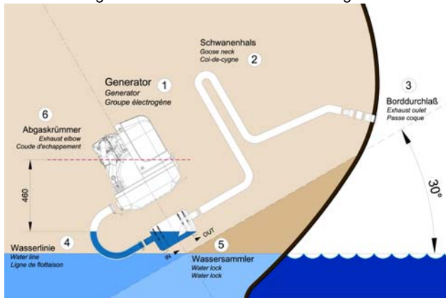
Fig. E.6.5.1-3: Position inclinée de 30 degrés
