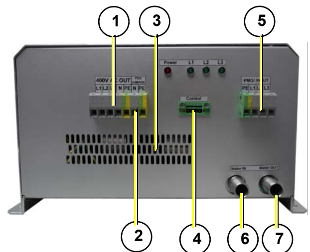
Fig. I.4-1: Côté raccordement
