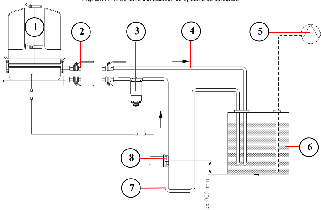
Fig. E.7.1-1: Schéma d'installation du système de carburant
