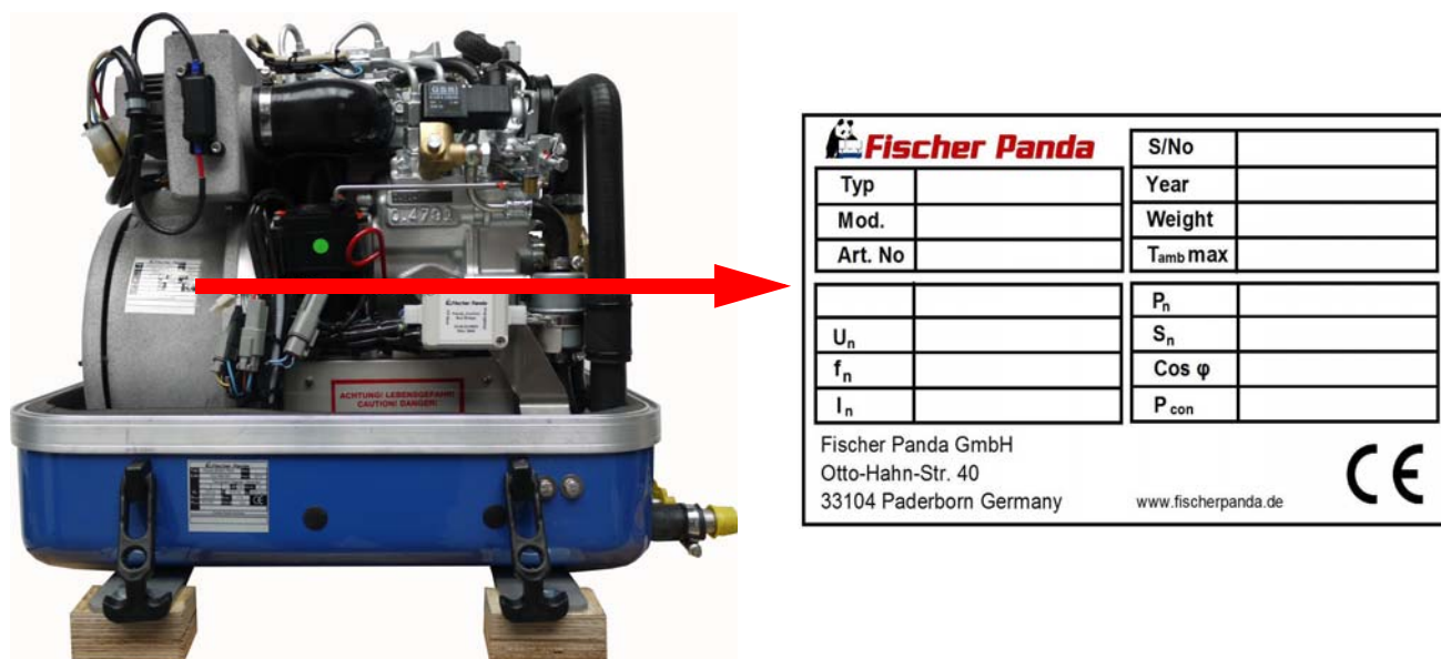
Fig. D.1-2: Description de la plaque signalétique
