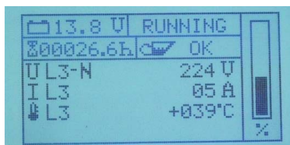
Fig. K.3.3.4-7: Tension simple L3
