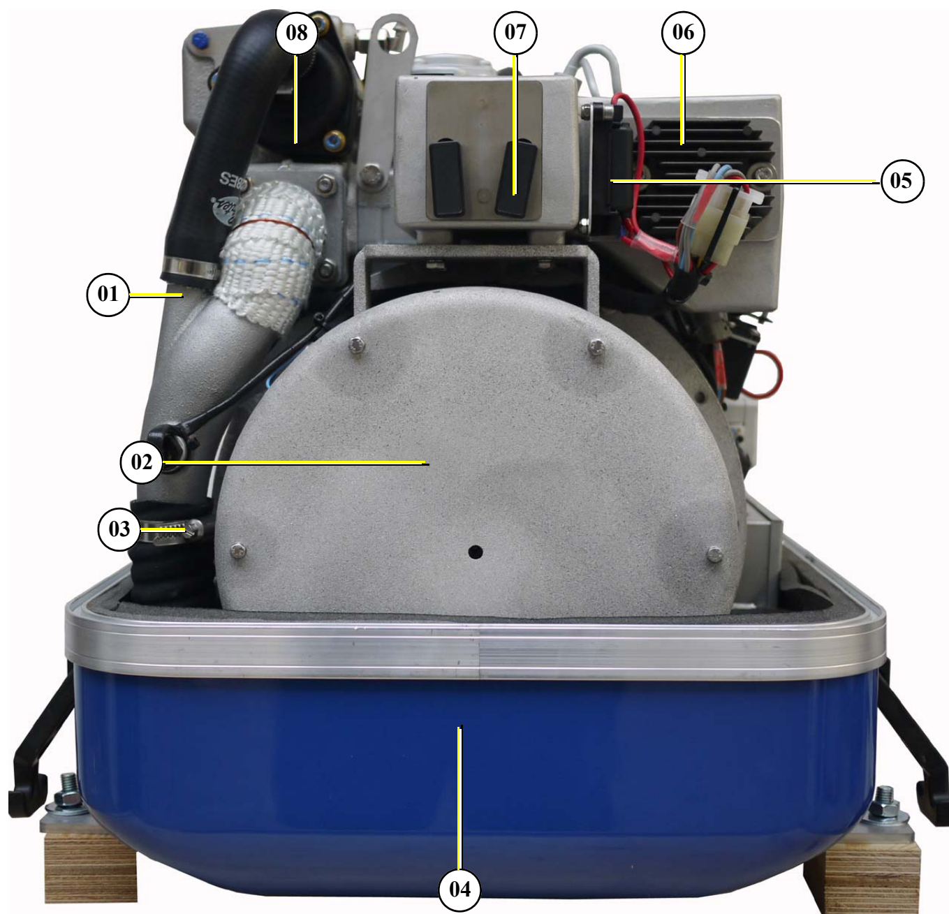
Fig. D.2.4-1: Vue arrière
