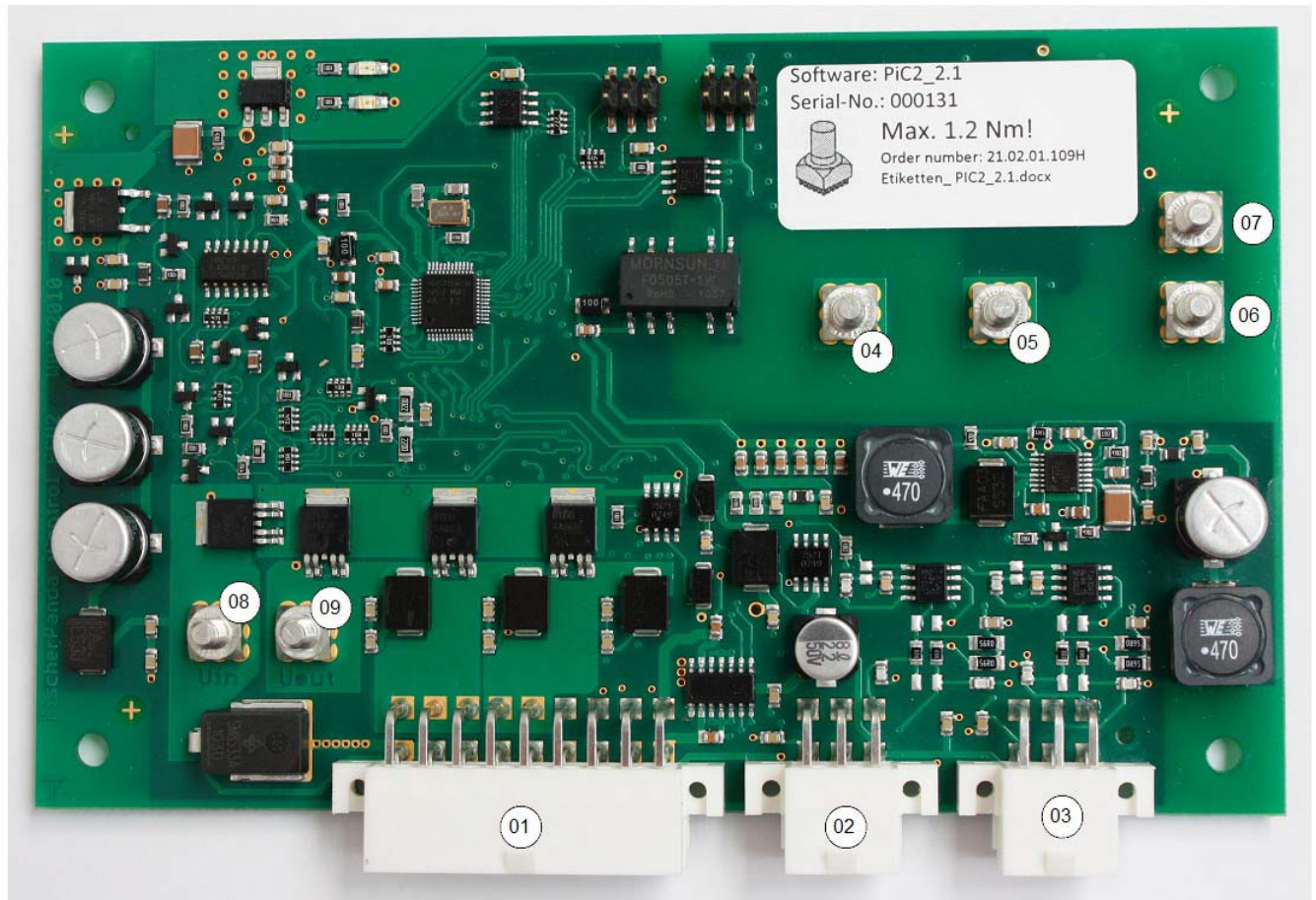
Fig. L.4-1: Branchements de la platine de commande Panda iControl
