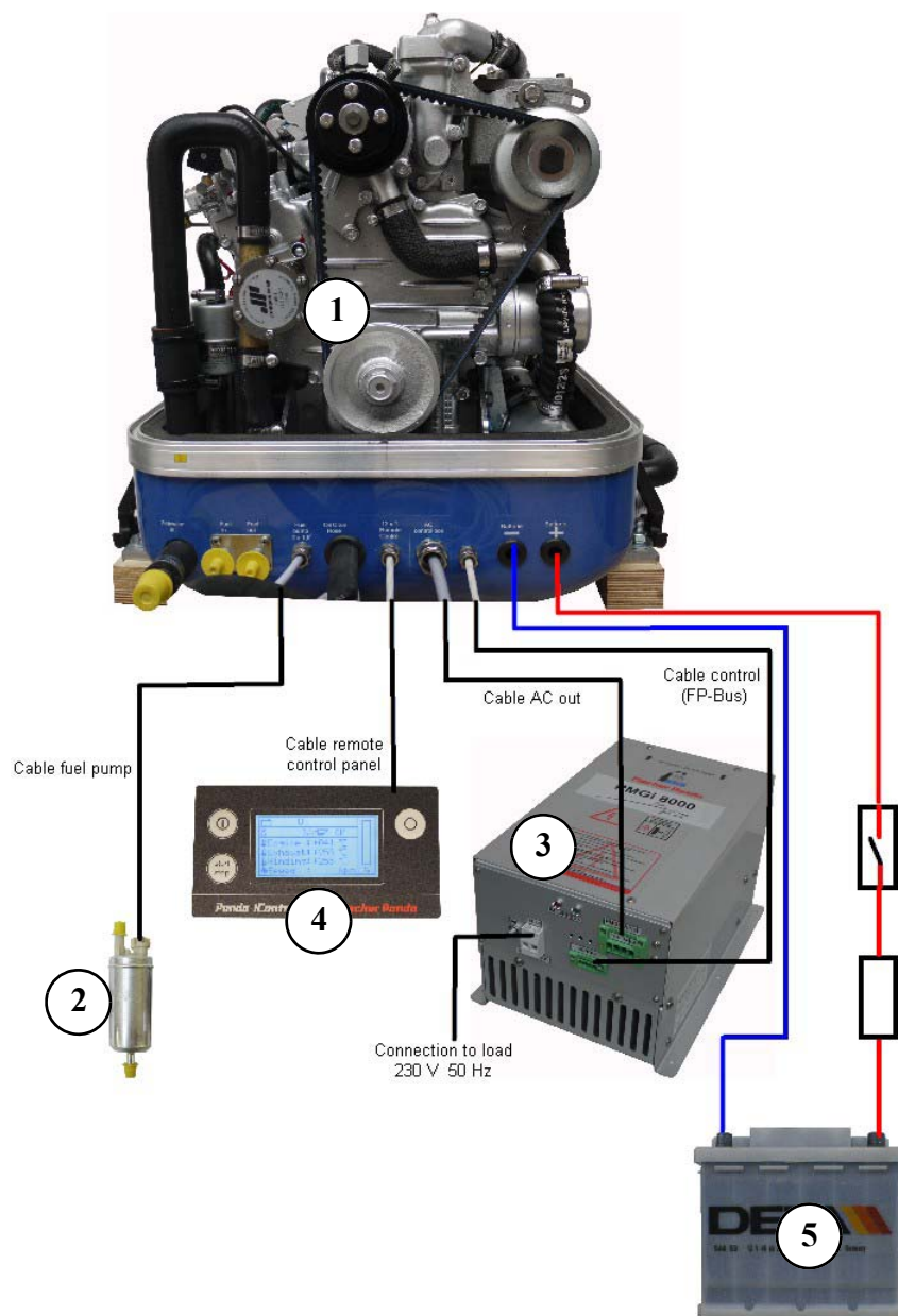
Fig. E.10-1: Installation électrique - Exemplel
